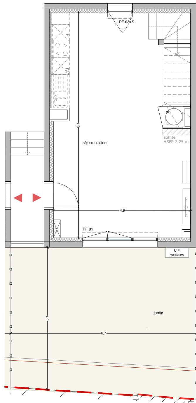
PLAN NIVEAU RDC
